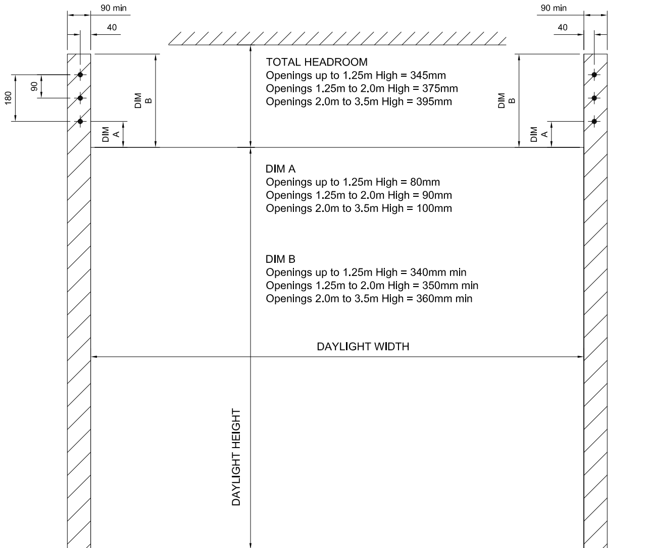
BACK FIX GUIDE
