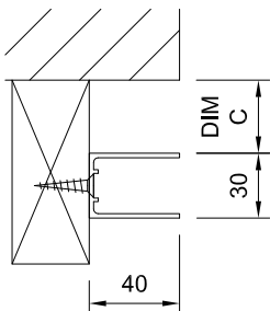
BACK FIX GUIDE
