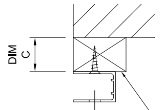
FACE FIX GUIDE
